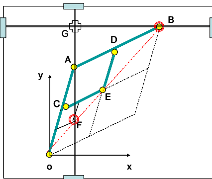
图 9 符合要求的装置示意图
