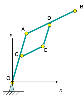
图 8 放大装置的原理图
