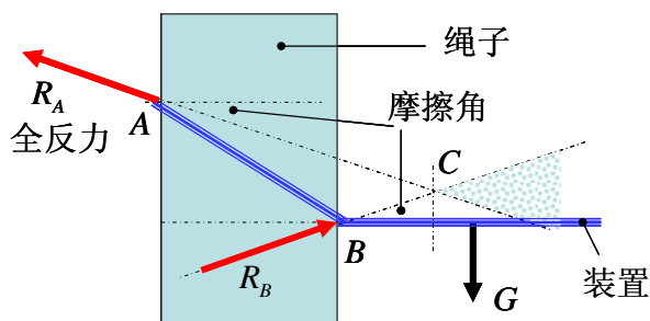
图 4 装置保持静止的条件
